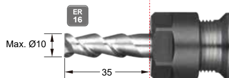
Vollhartmetall - Schaftfräser
