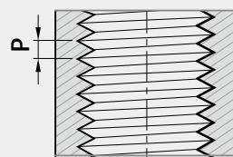
55° Paralleles Rohrgewinde 60° Paralleles Gewinde
