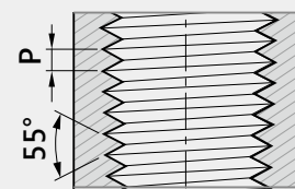
55° Kegeliges Rohrgewinde
